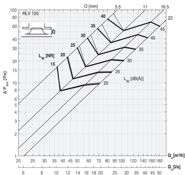
Charakteristika tlak-objemový průtok přiváděného vzduchu
