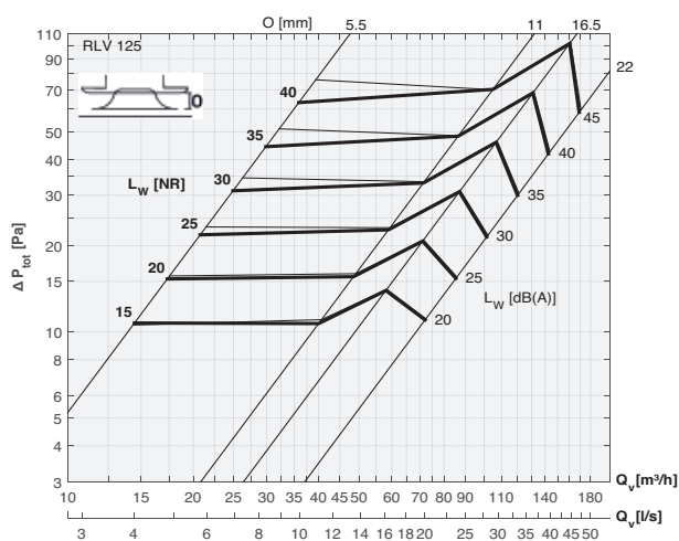
Charakteristika tlak-objemový průtok odváděného vzduchu
