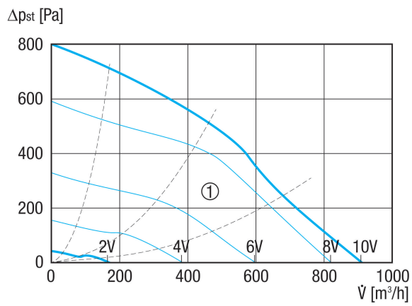
① Pomoćne krivulje za upravljački napon 2 - 10 V
