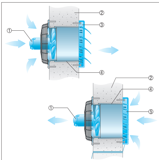
① Ventilátor
