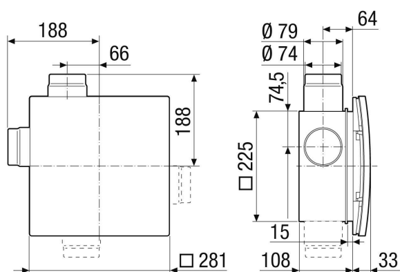
Rysunek wymiarowy [mm]
