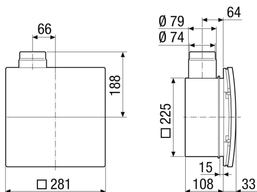
Rysunek wymiarowy [mm]
