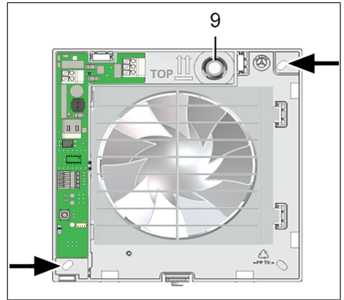
9 Cable grommet
