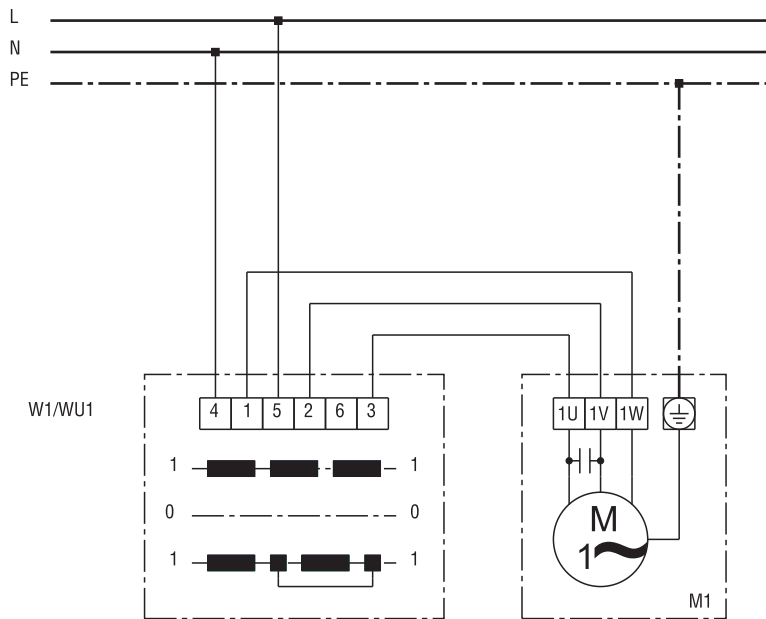
W1 / WU1 - Реверсивный переключатель: Вытяжная вентиляция / ВЫКЛ. / Приточная вентиляция M1 - Вентилятор (конденсаторный двигатель)
