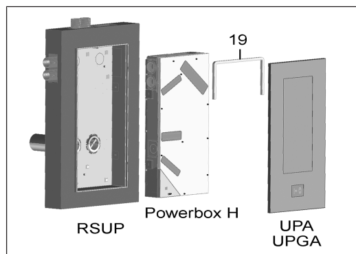
19 Bande d'étanchéité, élastique (dans la fourniture WS 75 UPA/UPGA)
