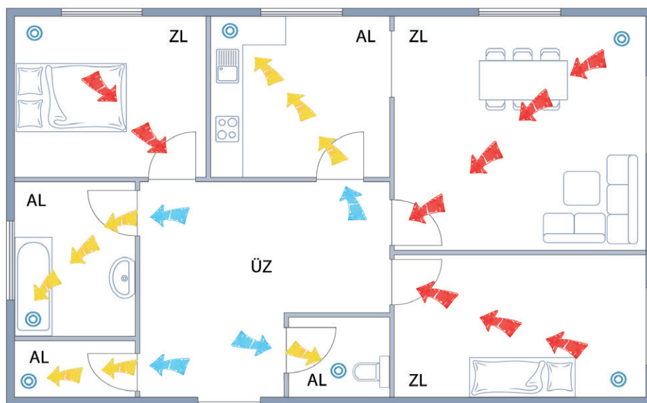
AL: Prostorija za odsisni zrak ZL: Prostorija za dobavni zrak ÜZ: Prestrujno područje
